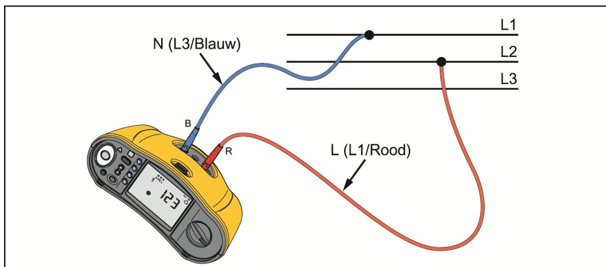
Afbeelding 7. Meting aan 3-fasig systeem
