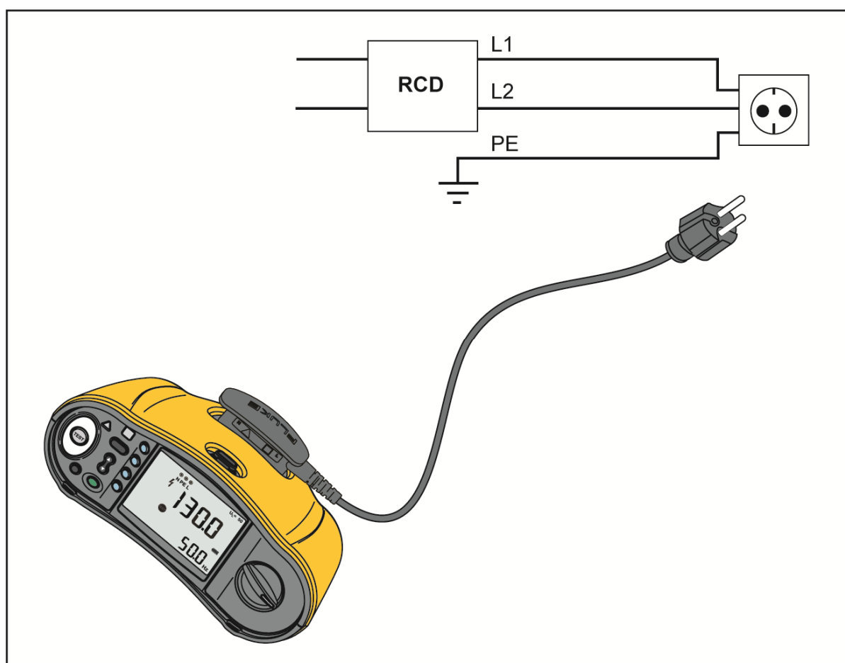
Afbeelding 12. Configuratie met enkel meetsnoer
