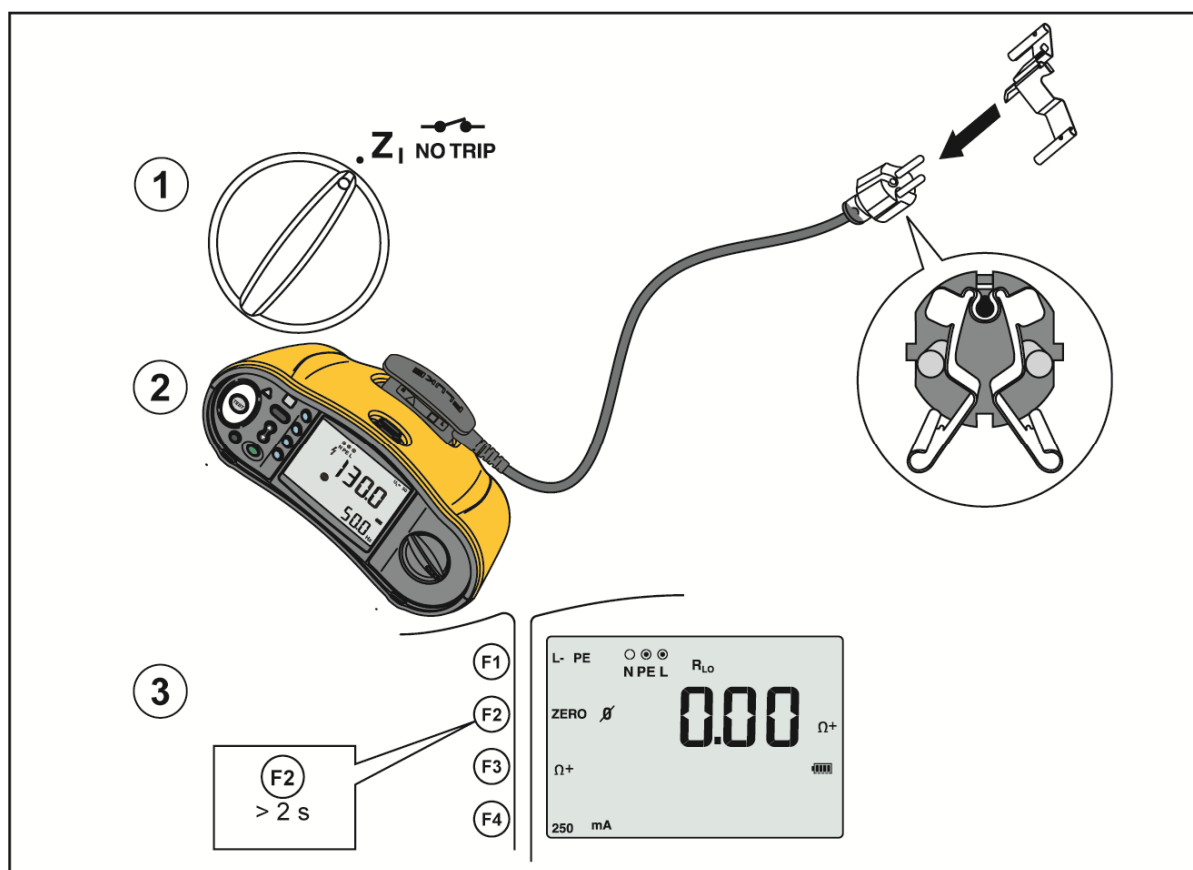
Afbeelding 2. Nulstellingsdisplay
