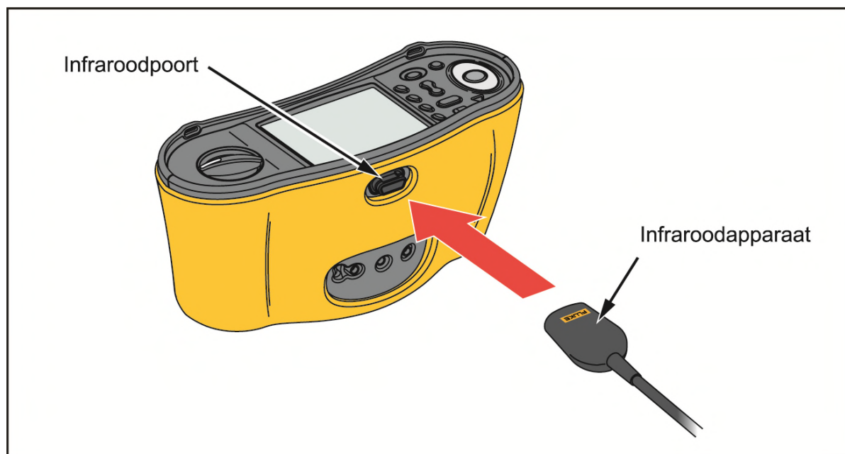
Afbeelding 19. Seriële IR-kabel bevestigen
