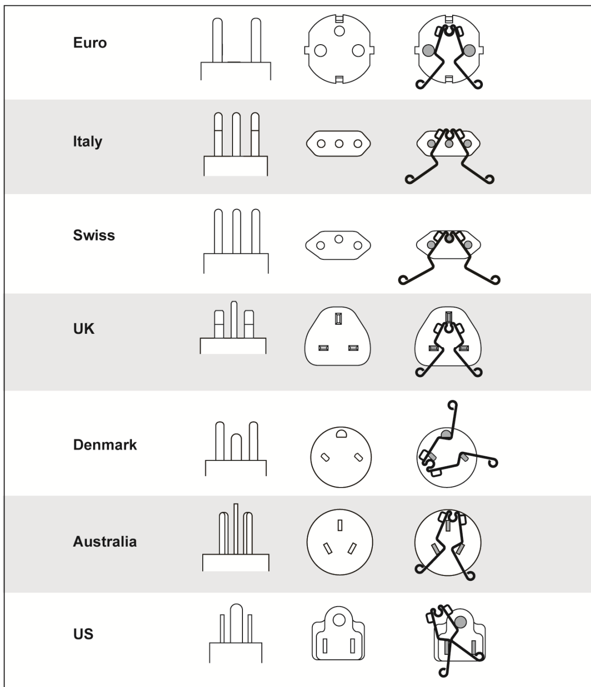
Afbeelding 3. Landspecifieke configuraties van de nulstellingsadapter
