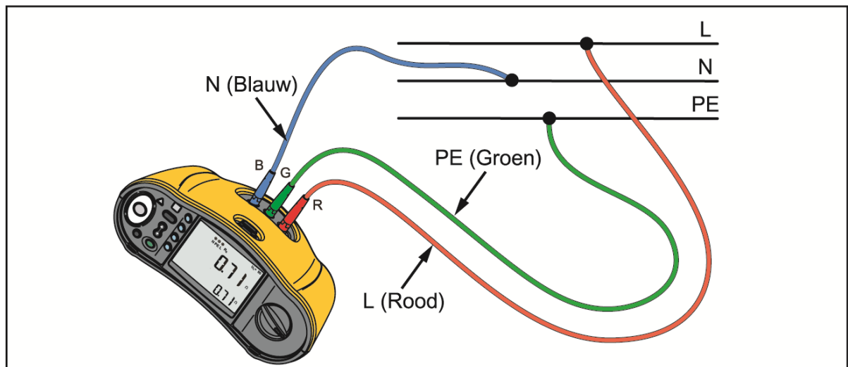
Afbeelding 4. Aansluitingen voor voorafgaande veiligheidstest
