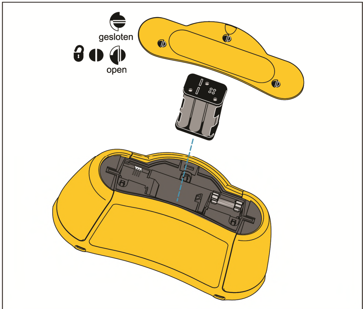
Afbeelding 20. Batterijen vervangen
