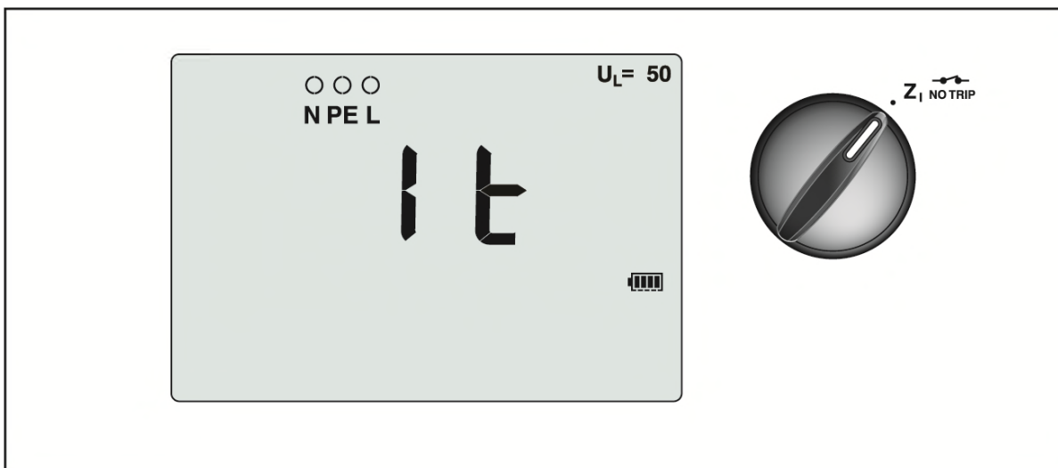
Afbeelding 6. Lusimpedantietest in IT-systeem
