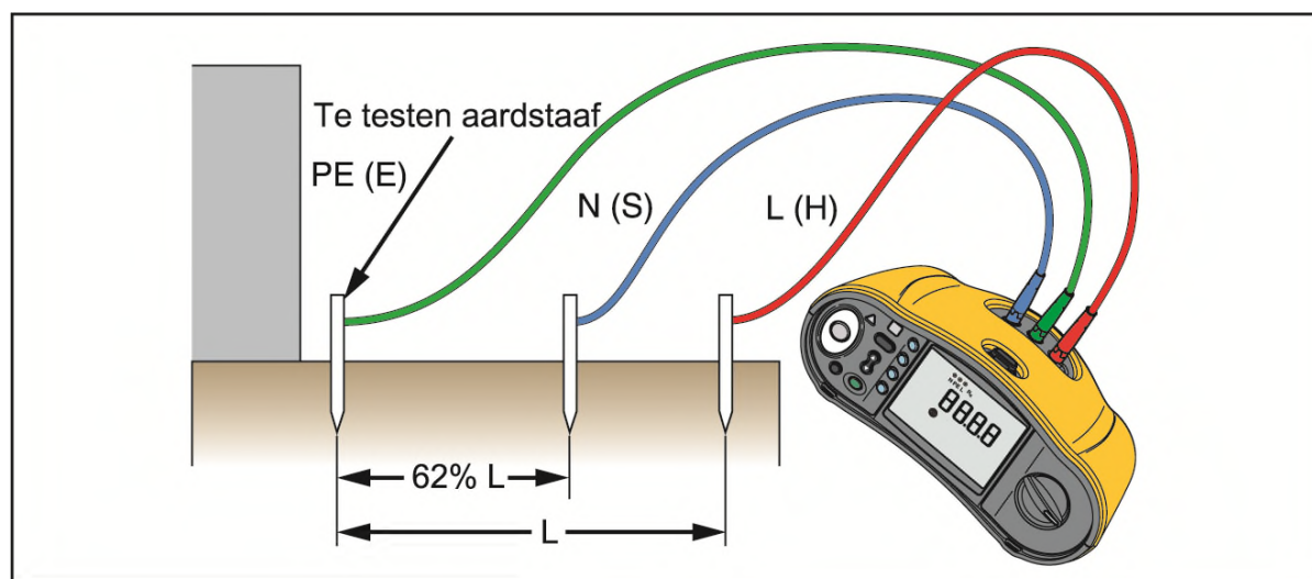
Afbeelding 15. Aansluiting voor aardingsweerstandtest
