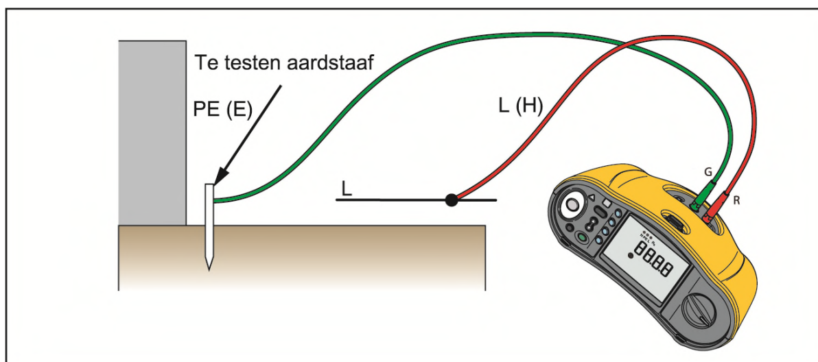
Afbeelding 17. 2-draads aansluiting voor lustest van aardsweerstand (hogestroom-tripmodus)
