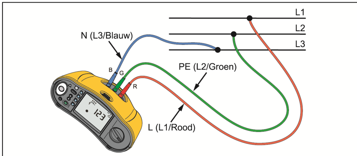
Afbeelding 13. Aansluiting voor faserotatietest
