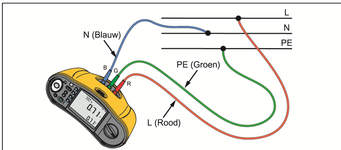
Afbeelding 16. 3-draads aansluiting voor lustest van aardingsweerstand (no-trip-modus)
